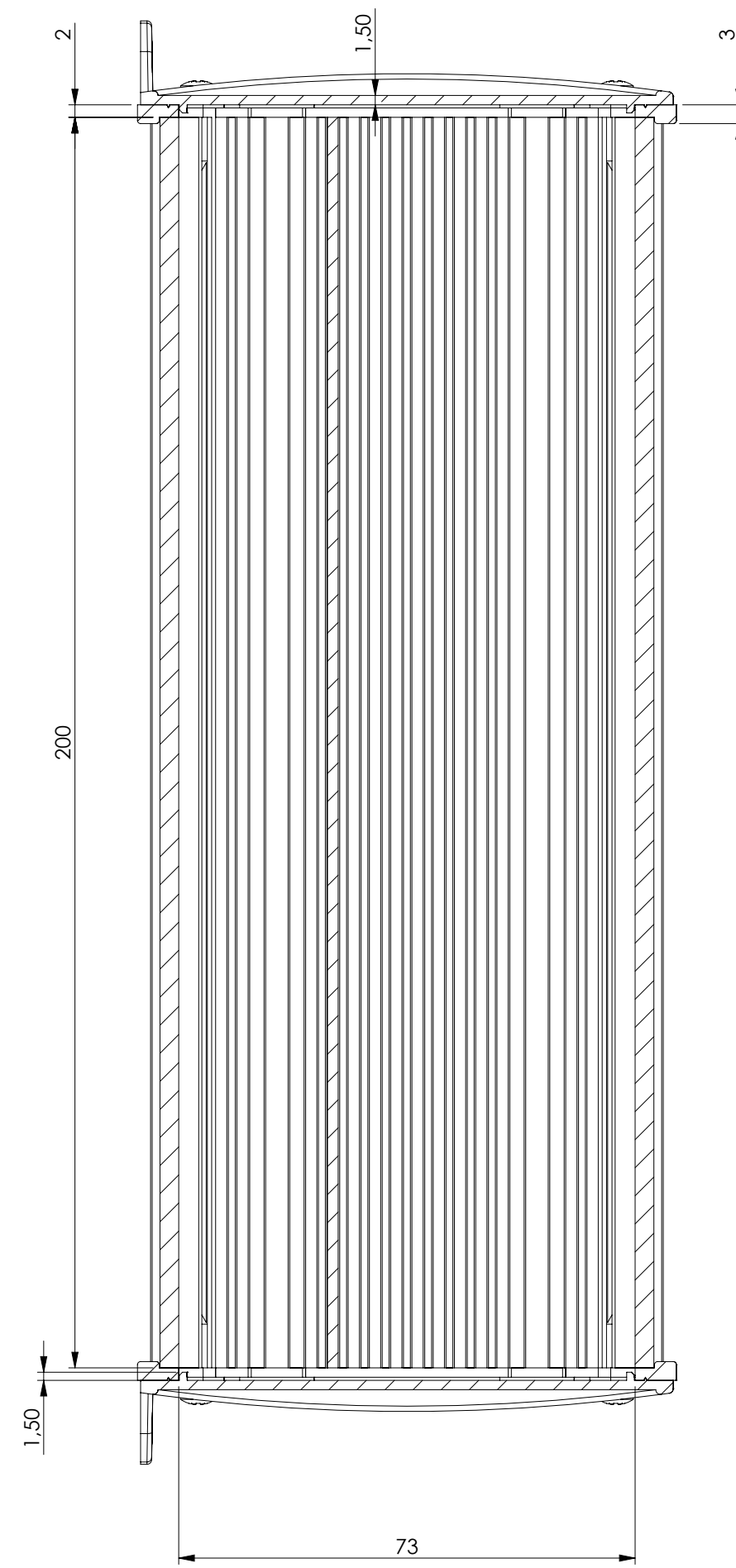
SEZIONE B-B
